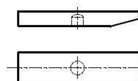
Forma J Nuožulnių kraštu ir grioveliu užfiksavimui with chamfer spring dowel sleeve
