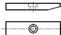
Forma G Nuožulnių kraštu ir viena skylė varžtui with chamfer and hole for retaining screw
