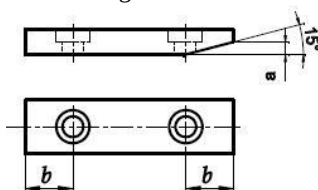
Forma H Nuožulnių kraštu ir dviem skylėm varžtui with chamfer and holes for 2 retaining screw
