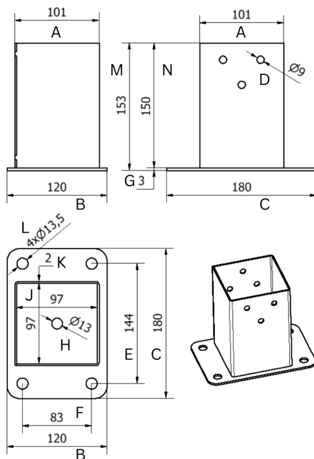
Matmenys/ Dimensions mm
